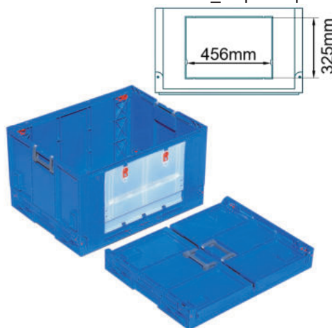
Bac avec portes latérales Réf. 9625_ déplié et plié
